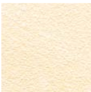
NÉALITE
