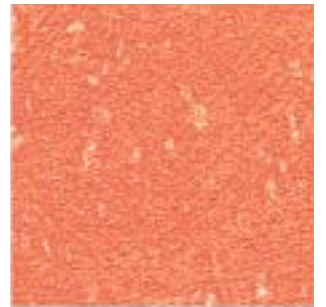
CÉRIUM
