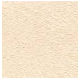
SABLÉ
