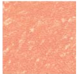
HÉMATITE
