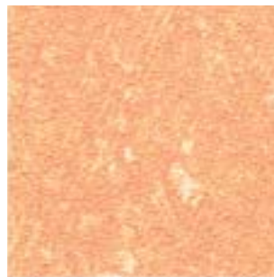
DOLOMITE
