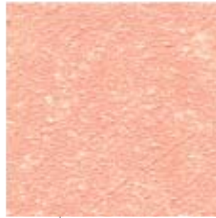
CINABRE
